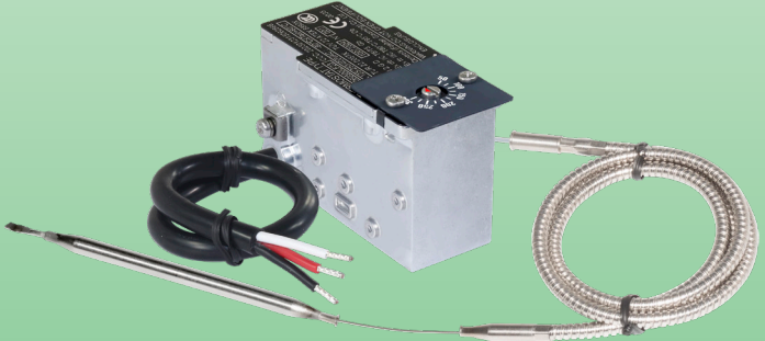
Thermostat Typ KAC mit 66CP01 bedrucktem Zifferblatt, montiert mit 2 M4-Schrauben
