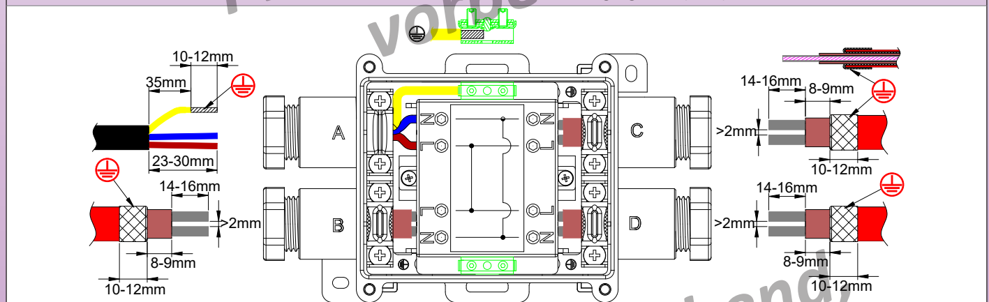
Modell mit 3 Heizdrähten und einem Stromversorgungskabel (YB14)
