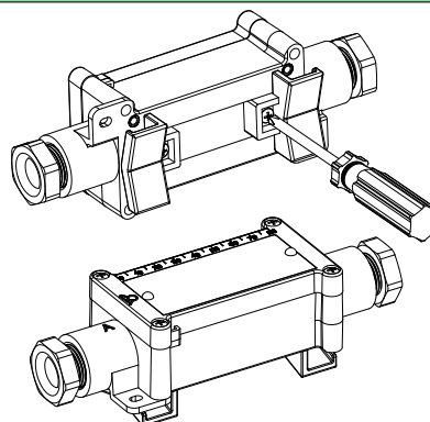
Beispiel für die Montage an einem Y40-Anschlusskasten für Begleitheizungen
