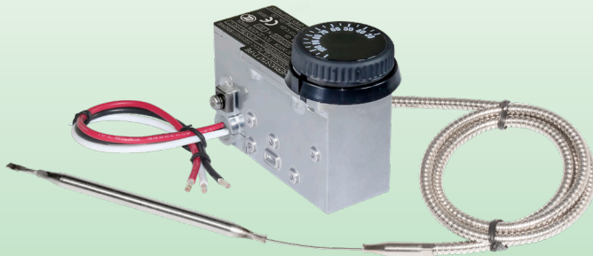
Thermostat Typ KAA mit Weichgriff-Knopf 66MZ und 66EN1 Blende
