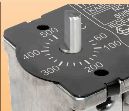
A: Schaft, Ø 6mm, Länge 10mm, zur Verwendung mit bedruckten Knöpfen und Blenden oder kleinen Kunststoff-Pfeilknöpfen (als Zubehör unten erhältlich)
